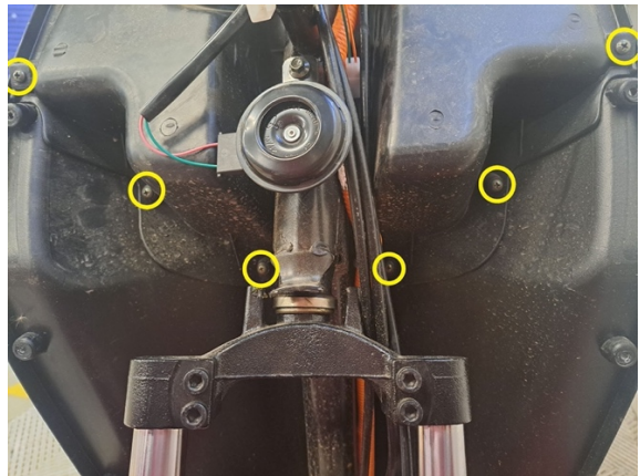
Irrota etukatteen alemman sisäosan kiinnitysruuvit. (ristipäämeisseli ph2).
